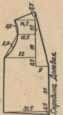
Полочка жилета 2 дет.
