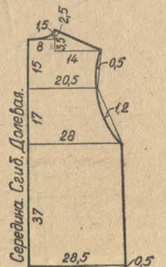
Спинка жилета 1 дет.
